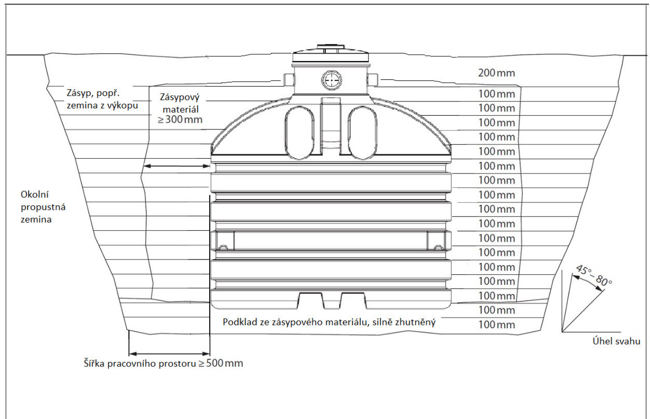
Obr. 4: Provedení montáže na příkladu podzemní nádrže Oasis 6000 litrů s poklopem nádrže Basic
